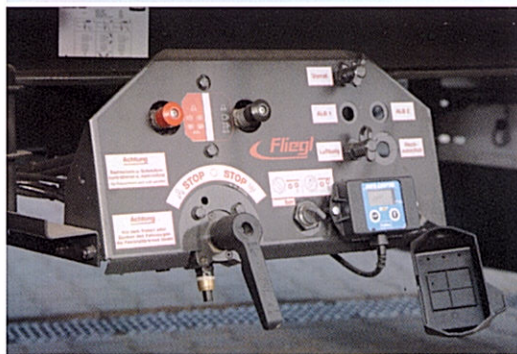
Fácil y visible manejo. Nuestro cuadro de manejo y mantenimiento está valorado por la prensa del transporte
