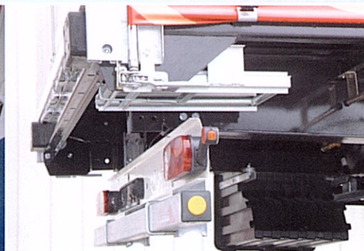
Parachoques y soporte para luces están disponibles como componentes separados, de tal manera que en caso de avería sea económico y fácil de sustituir.
