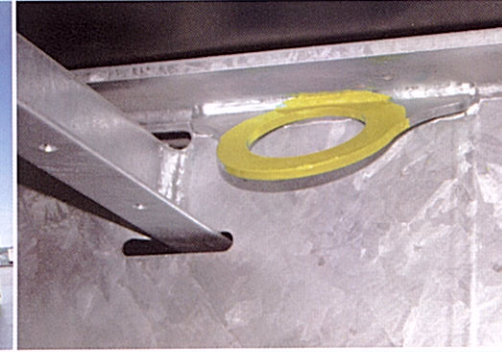
Las anillas de amarre de barco hacen posible tensar el semirremolque de manera segura y fiable para el transporte naval, incluso sin tractora.
